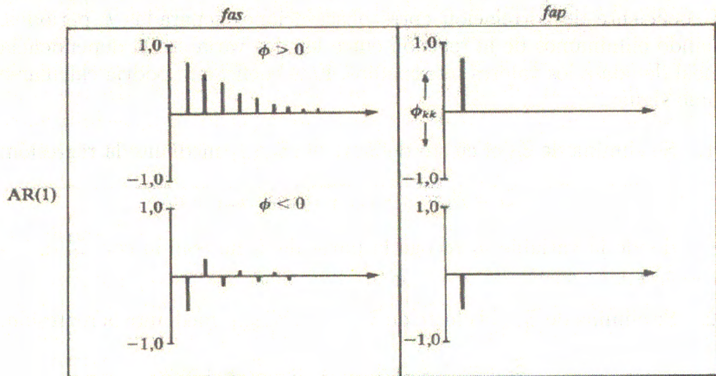
Figura 4.7 Funciones de autocorrelación simple y parcial para procesos AR
