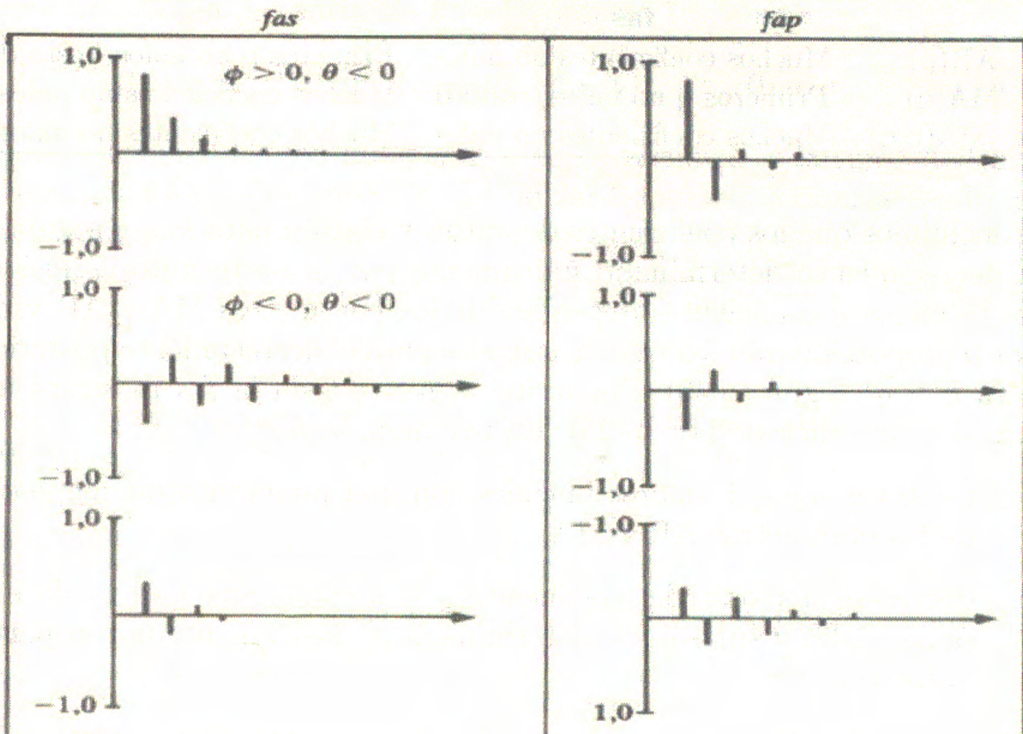
Figura 5.7 Funciones de autocorrelación simple y parcial para procesos ARMA(1,1)
